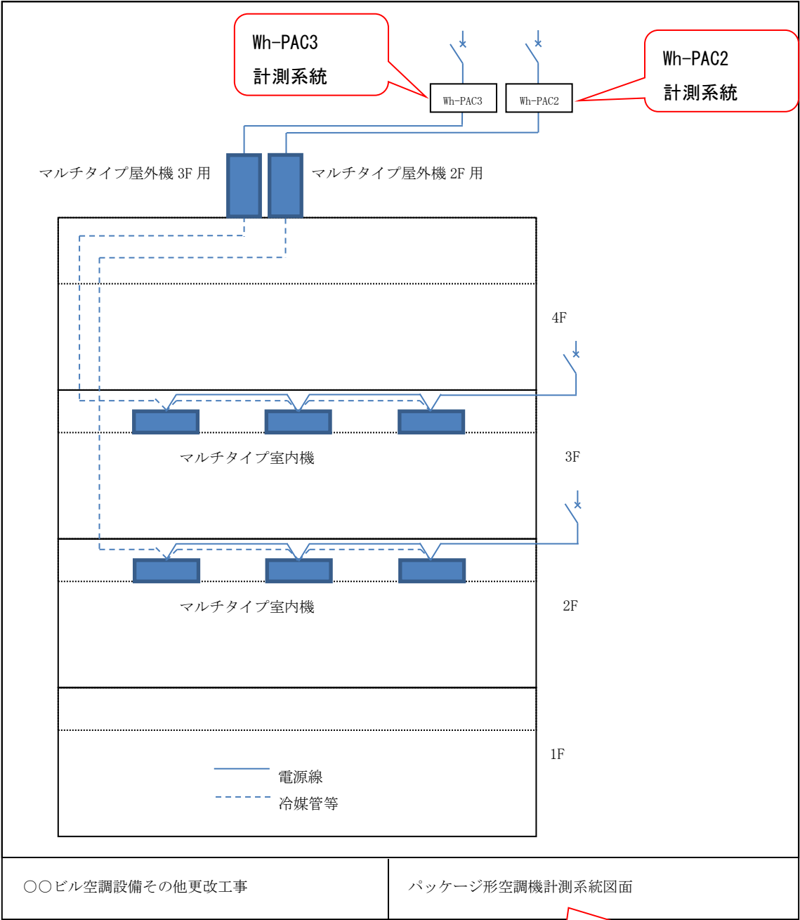
計測系統を示した図面例：高効率パッケージ形空調機の導入
