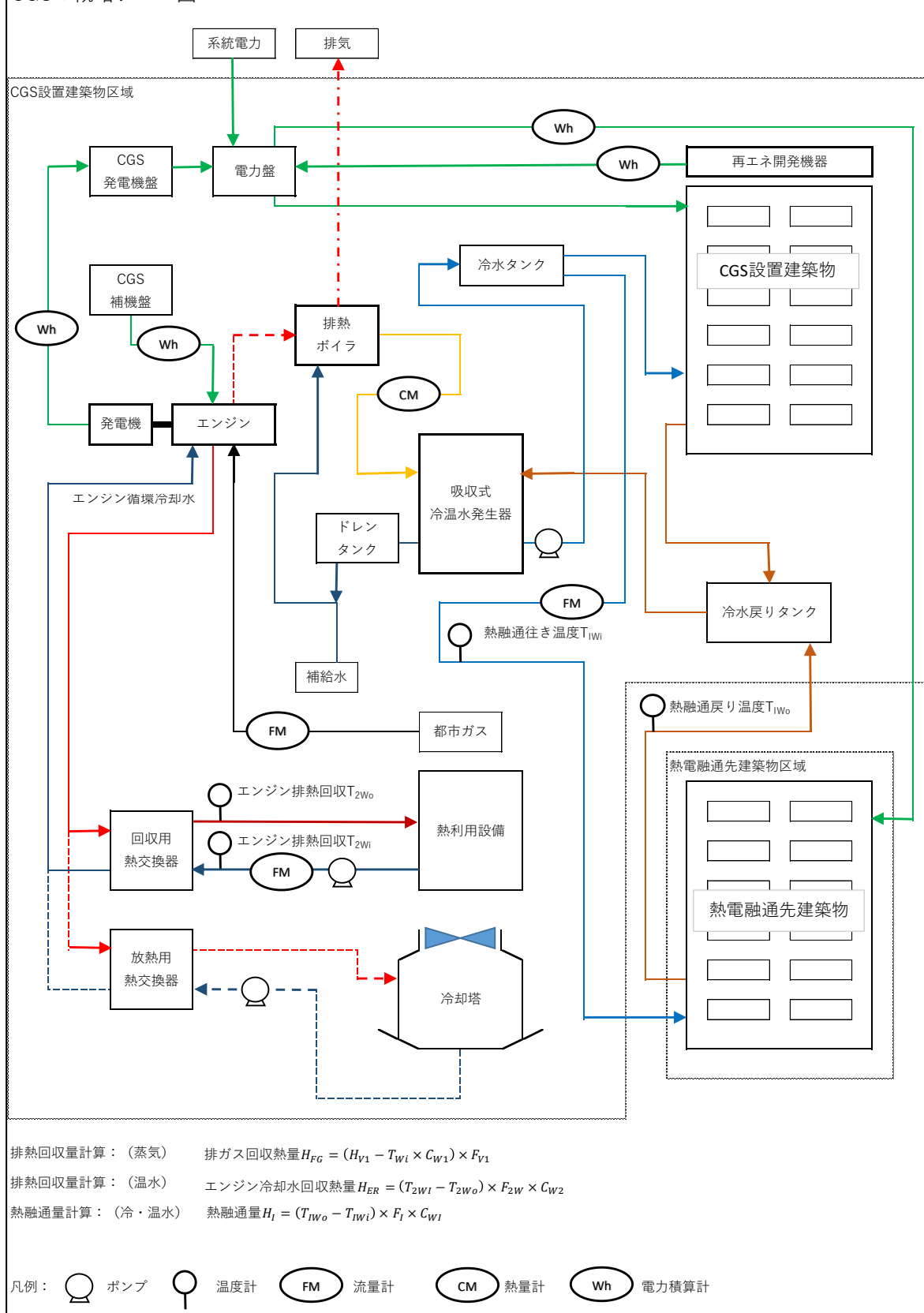
CGSの概略フロー図
