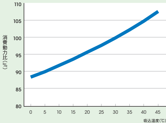
図Ⅲ-7-3 コンプレッサの吸込温度と消費動力の関係
