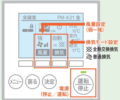
全熱交換器の操作盤の例 その3
