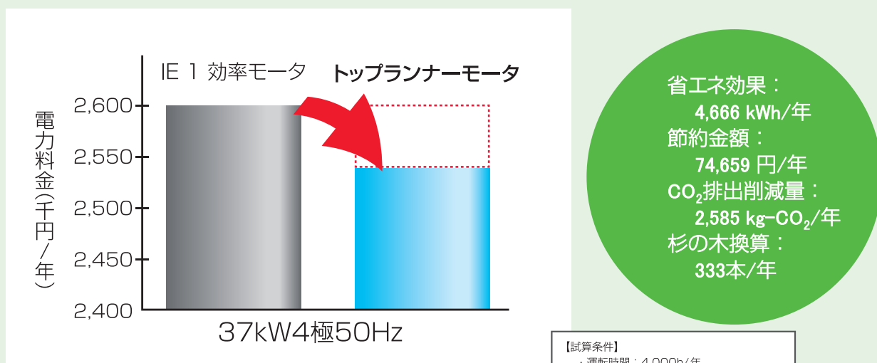
図Ⅲ-9-2 トップランナーモータの省エネ効果
