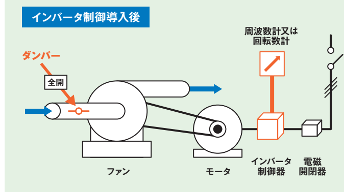
図Ⅲ-6-1 インバータ導入後の風量調整方法のイメージ
