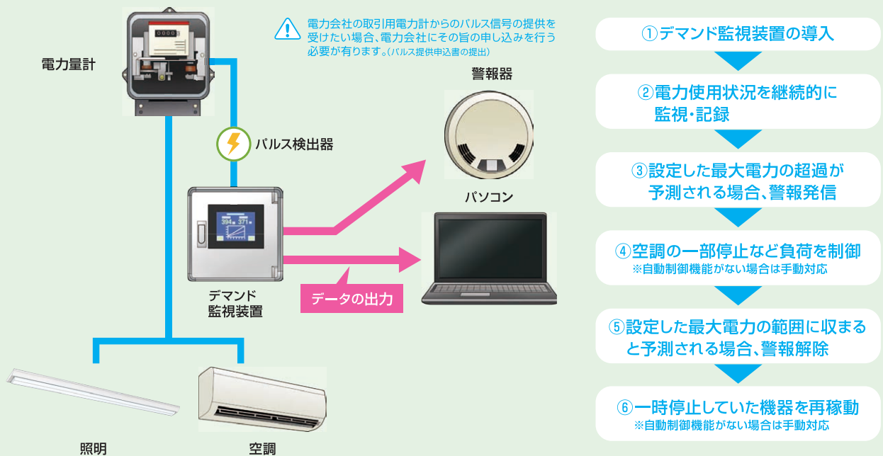
図Ⅲ-1-1 デマンド監視装置のイメージ
