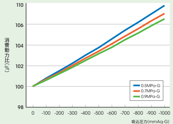
図Ⅲ-7-4 コンプレッサの吸込圧力と消費動力の関係
