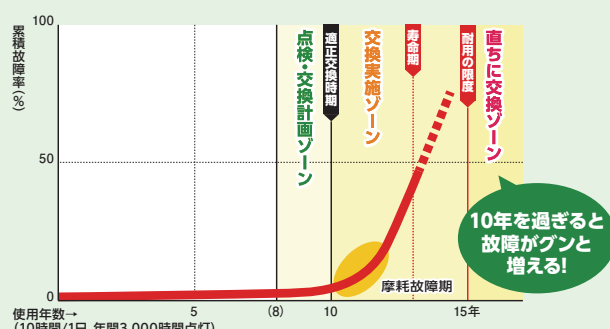
図Ⅲ-2-14 故障率と器具交換イメージ
