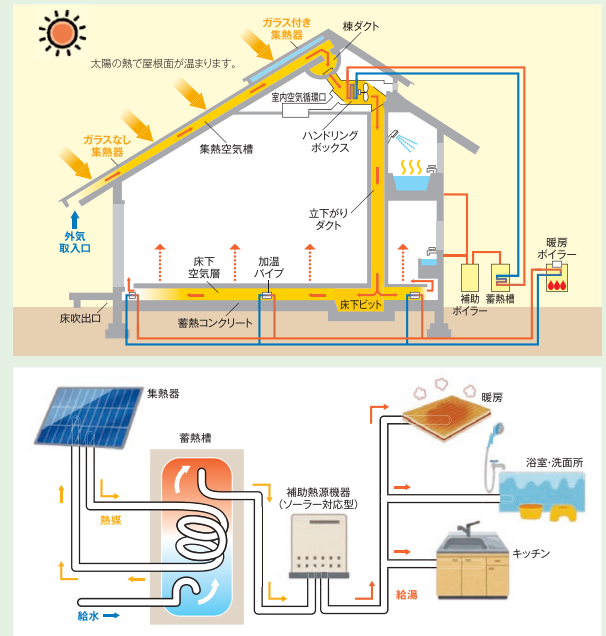
図IV-5-1 太陽熱利用システムのしくみ
