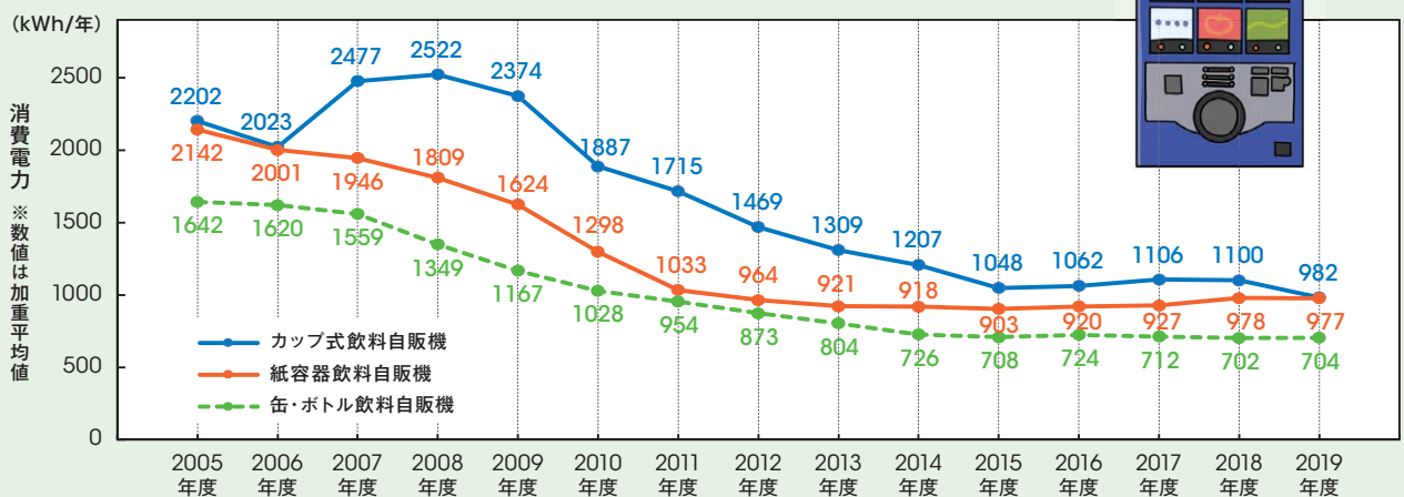
図Ⅲ-5-1 飲料自販機出荷台数1台あたりの年間消費電力(kWh)
