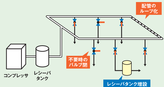
図Ⅲ-7-2 エア配管のイメージ
