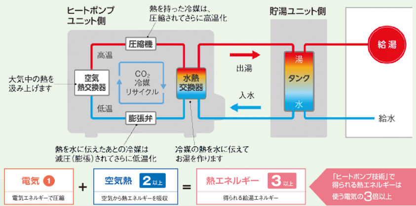
図Ⅲ-5-2 エコキュートの仕組み
