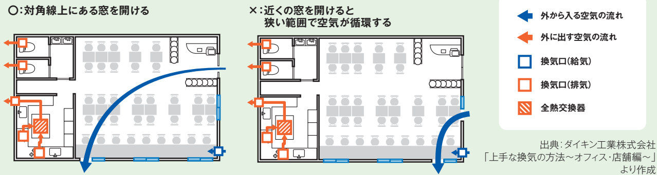
図Ⅲ-3-5 効率的な窓開けの例
