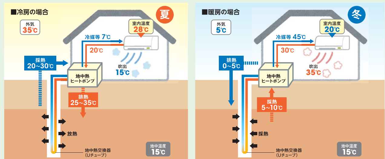
図IV-5-2 ヒートポンプシステムを活用した地中熱利用の例
