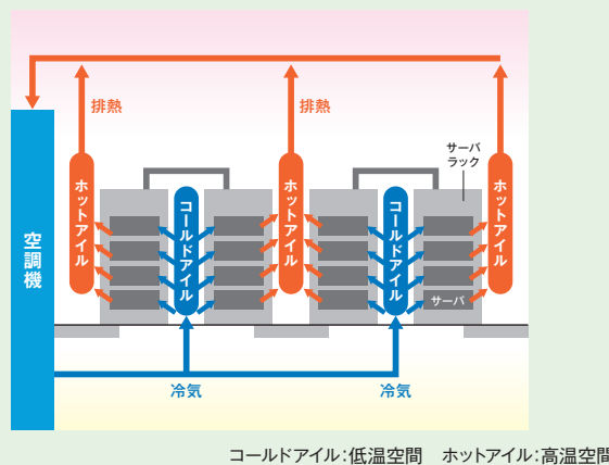
図Ⅲ-4-1 サーバ室空調システムの例
