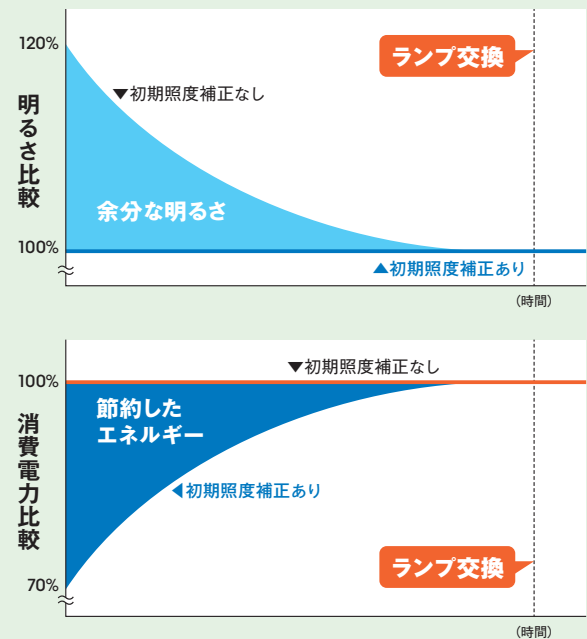
図Ⅲ-2-9 初期照度補正機能の効果
