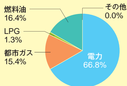
■ 都内CO 2 燃料種別排出量（2018年度実績）
