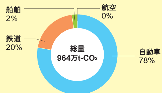
■都内運輸部門運輸機関別CO 2 排出量構成比 (2018年度速報値)
