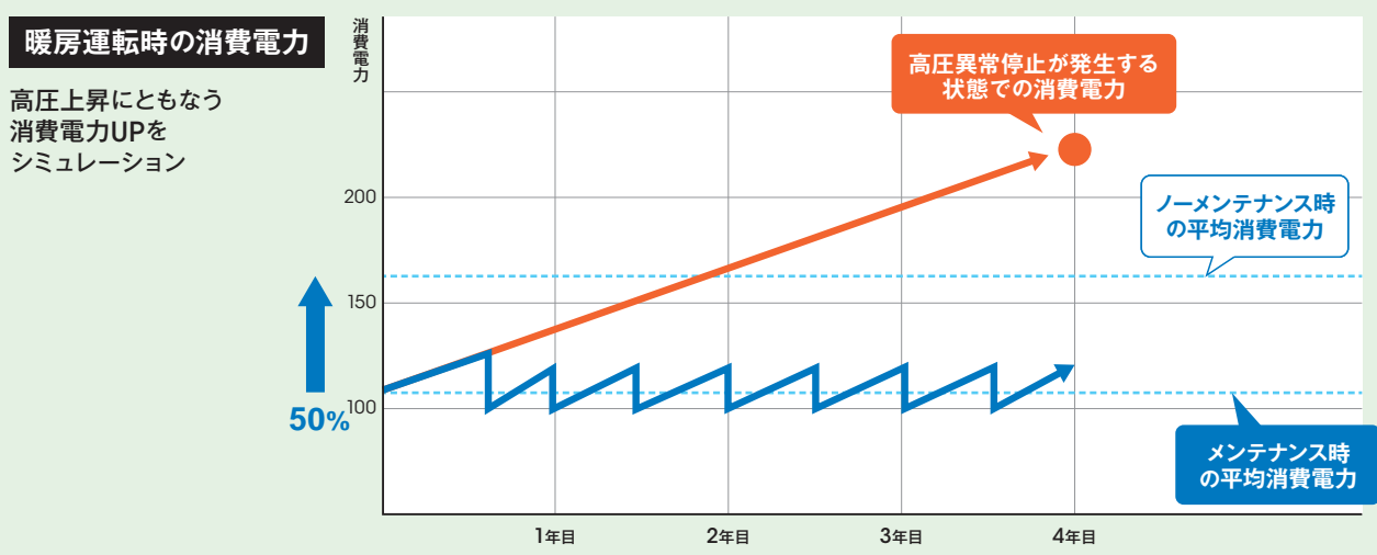
図Ⅲ-3-10 ノーメンテナンスによる消費電力の増加
