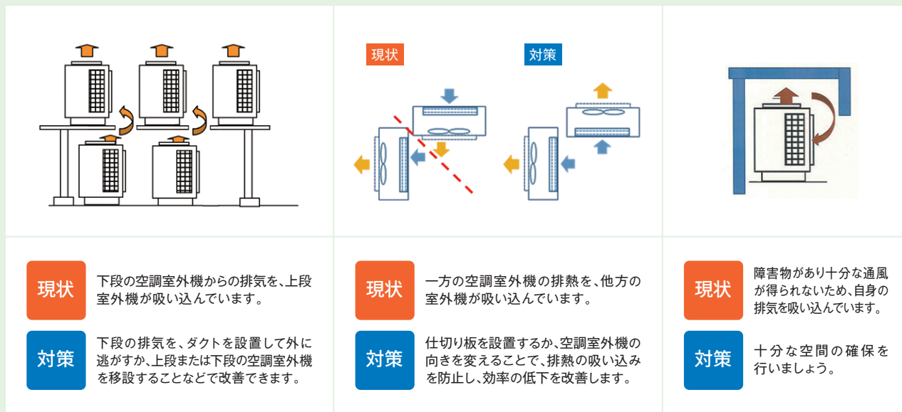
図Ⅲ-3-9 空調室外機周辺のショートサーキット防止対策
