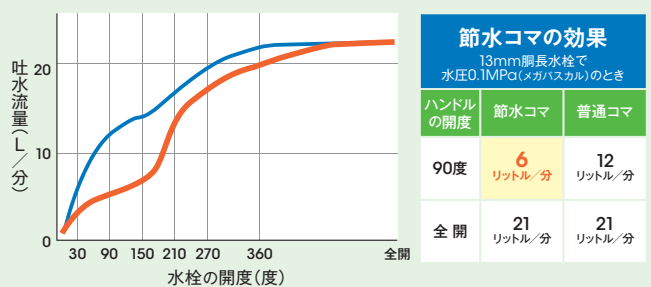
図Ⅲ-5-6 節水コマと普通コマの比較
