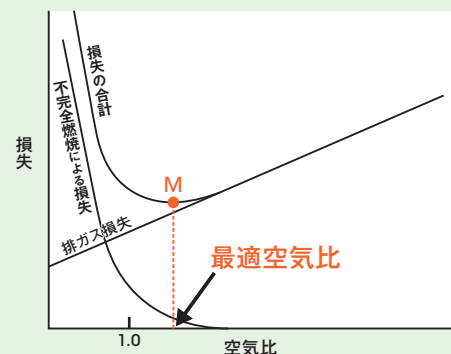
図Ⅲ-8-1 合理的な燃焼の状態
