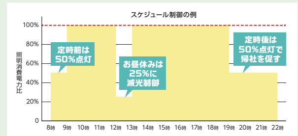
図Ⅲ-2-12 スケジュール制御の例
