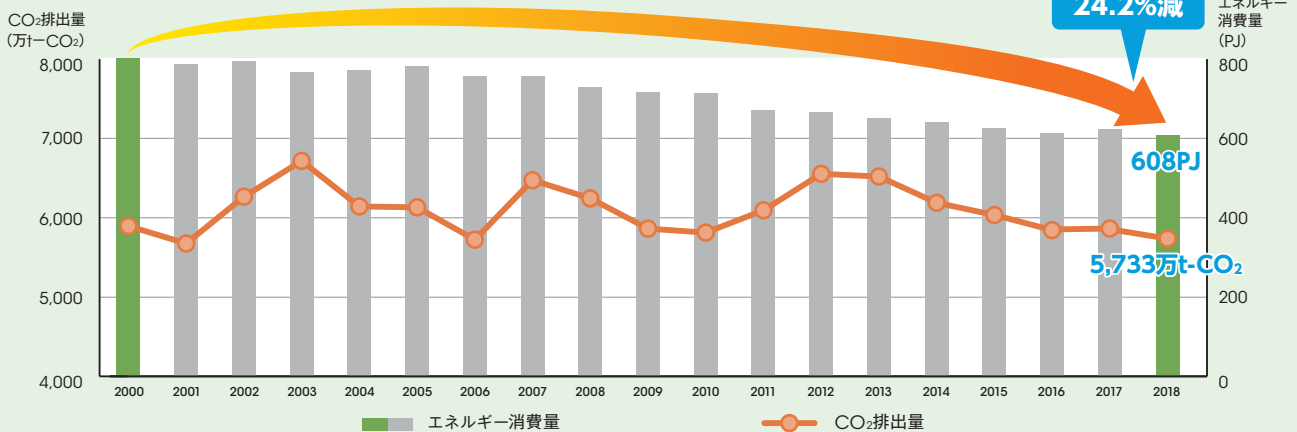
図I-3-1 東京都のエネルギー消費量及び総CO 2 排出量の推移
