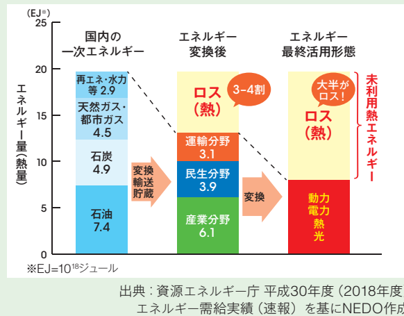
図Ⅲ-11-1 国内の一次エネルギー活用状況
