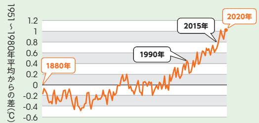
図 I-1-2 世界の平均気温の推移
