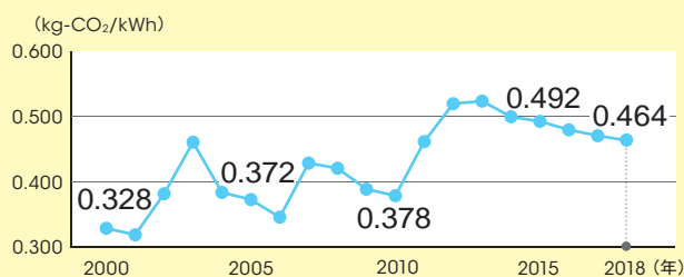
■ 都内に供給される電力のCO 2 排出係数※（推移）
