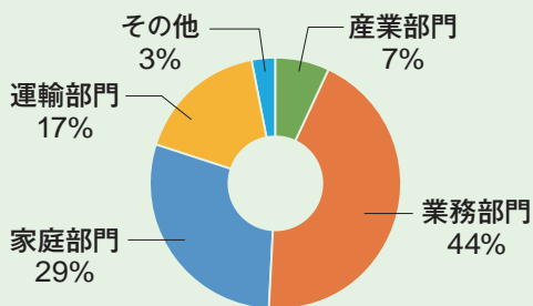
図I-3-2 東京都のCO 2 排出量の部門別構成比 (2018年度)
