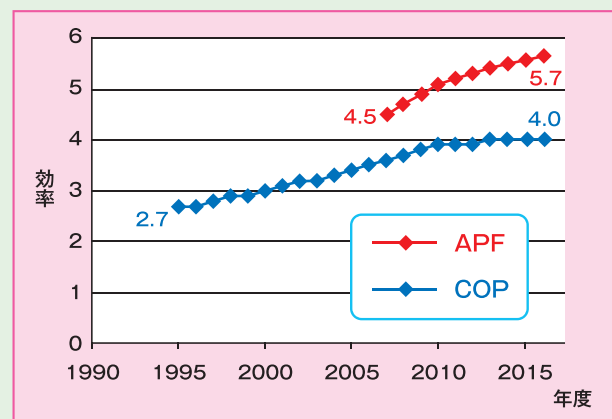
図Ⅲ-3-12 空冷パッケージ空調機の効率推移(28kWの場合)
