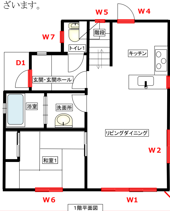
1階平面図
