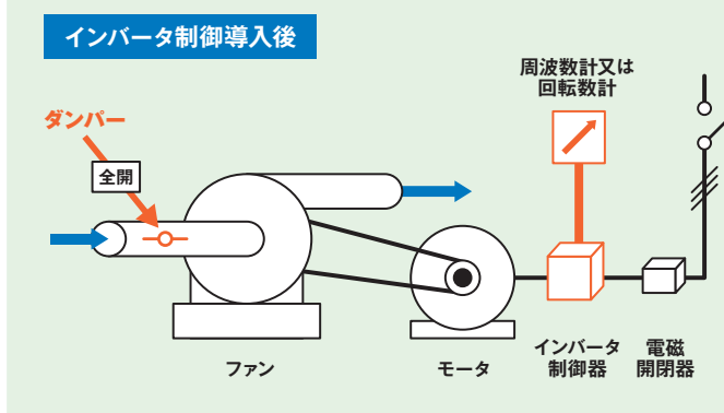
図Ⅲ-6-1 インバータ導入後の風量調整方法のイメージ
