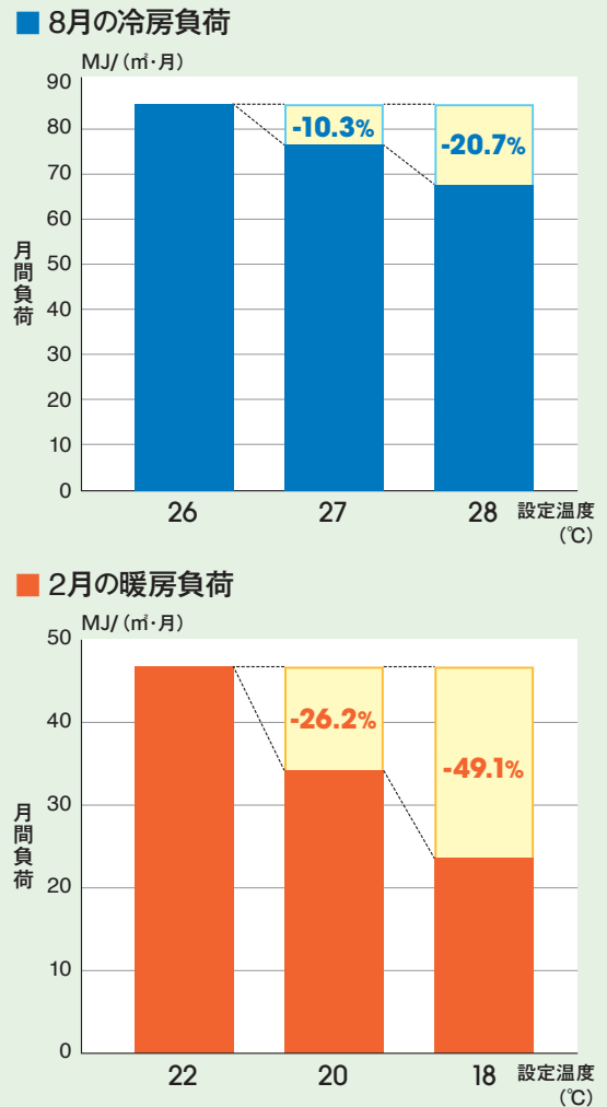
図Ⅲ-3-1 冷暖房設定温度と負荷
