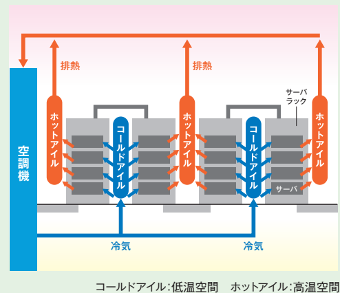
図Ⅲ-4-1 サーバ室空調システムの例
