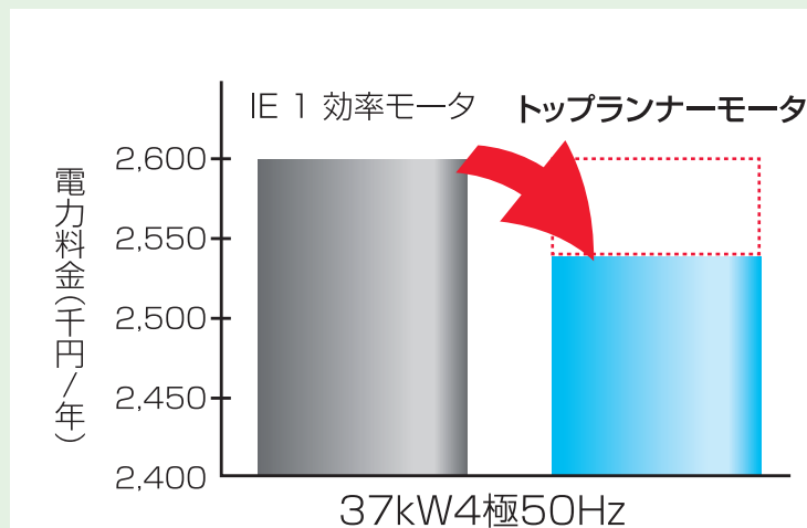
図Ⅲ-9-2 トップランナーモータの省エネ効果
