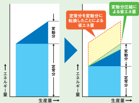
図Ⅲ-9-1 定常分と変動分の圧縮
