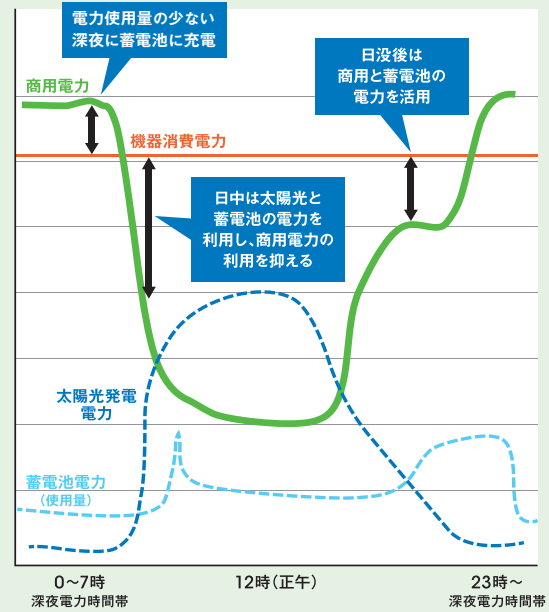
図Ⅳ-5-3 蓄電池と太陽光発電を活用した電力量抑制の例
