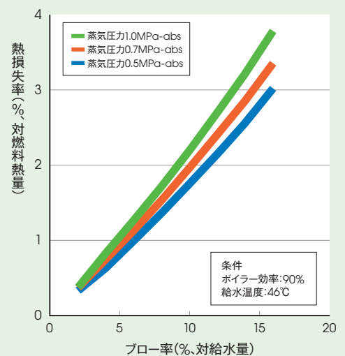
ブローによる熱損失率(熱回収しない場合)
