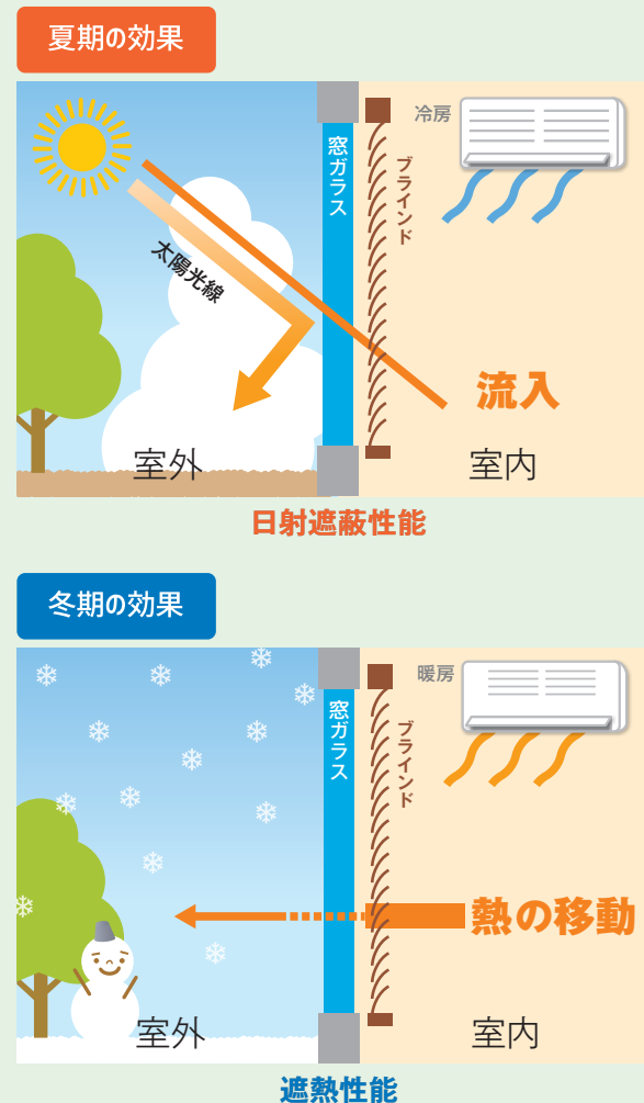
図Ⅲ-3-11 ブラインドによる省エネ効果
