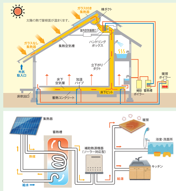
図IV-5-1 太陽熱利用システムのしくみ
