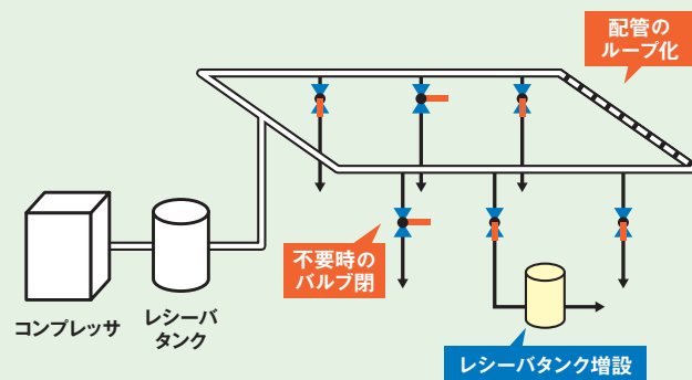
図Ⅲ-7-2 エア配管のイメージ
