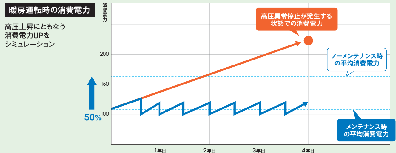
図Ⅲ-3-10 ノーメンテナンスによる消費電力の増加
