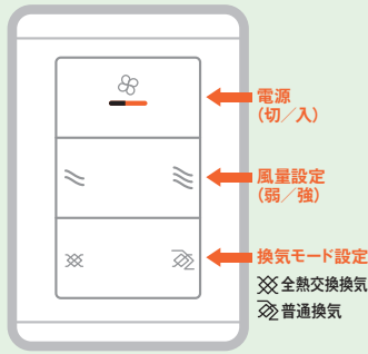
全熱交換器の操作盤の例 その2
