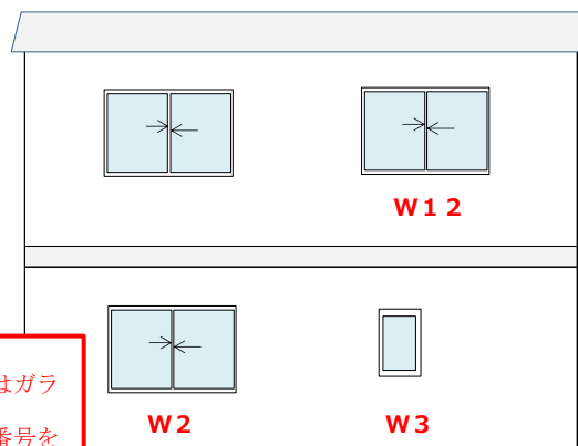
東側立面図
